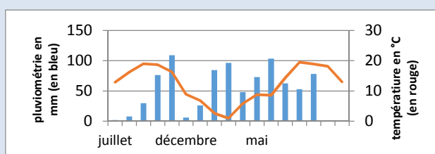
Pluviométrie et température mensuelles au Mourier
