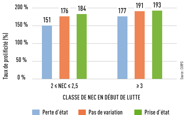
GRAPHIQUE 3 : Taux de prolificité des brebis en fonction de leur note d'état corporel en début de lutte et de la dynamique de NEC au cours de la lutte 2
