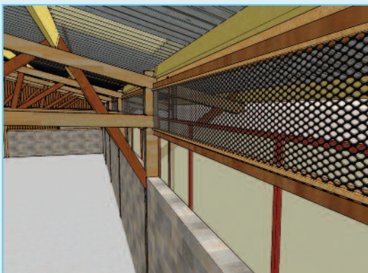
Figure 24 : Ventilation guillotine protégée (vue intérieure)
