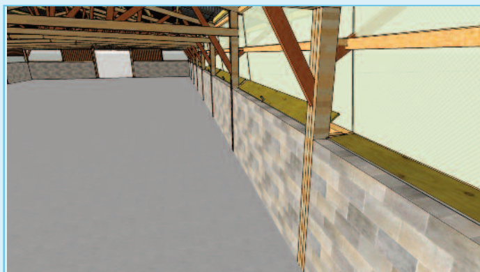
Figure 20: Ventilation bandeau décalé avec volets réglables (fermé et 45°) - solution initiale
