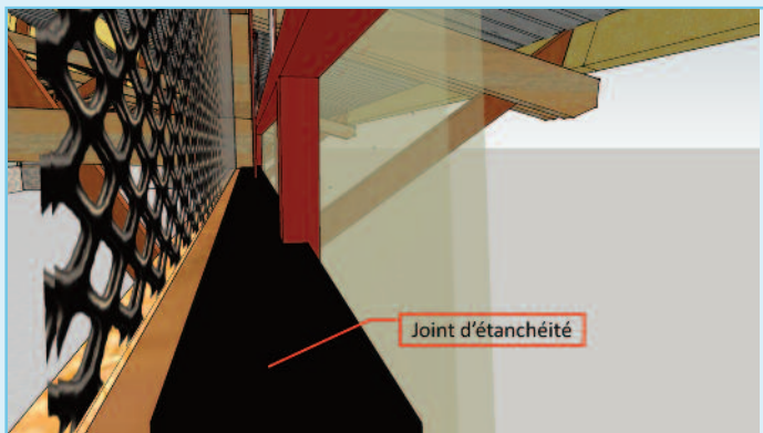
Figure 25 : Ventilation guillotine protégée (détail montrant le joint d'étanchéité)
