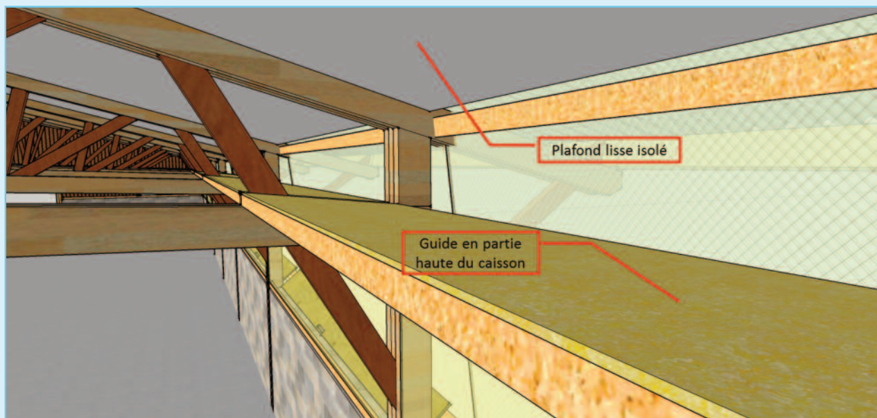
Figure 22: Bandeau décalé avec caisson translucide et guide sous rampant de toiture isolée
