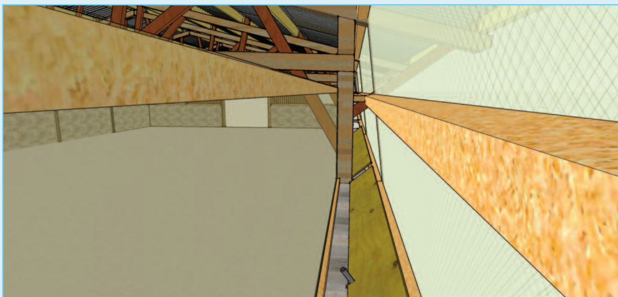
Figure 21: Bandeau décalé avec caisson translucide (pour éviter les courants d'air retombant sur les animaux)
